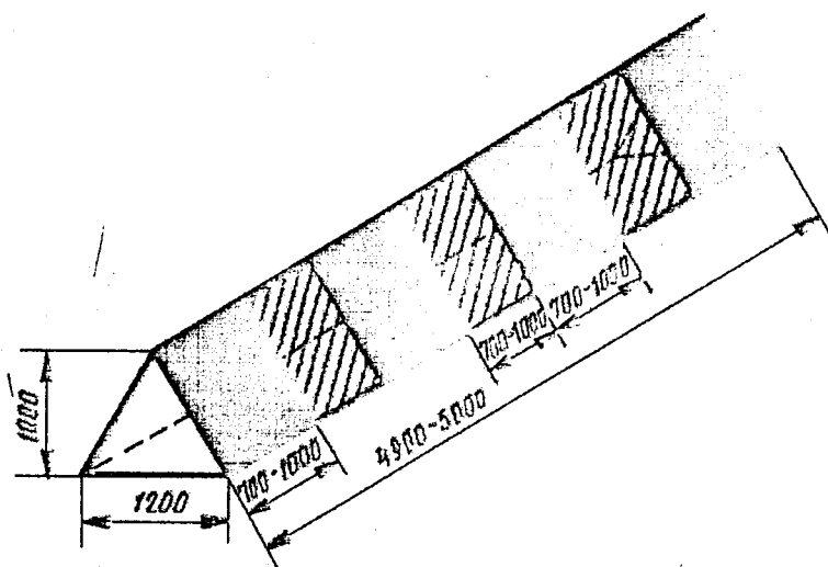
Рисунок. Входной маркер
